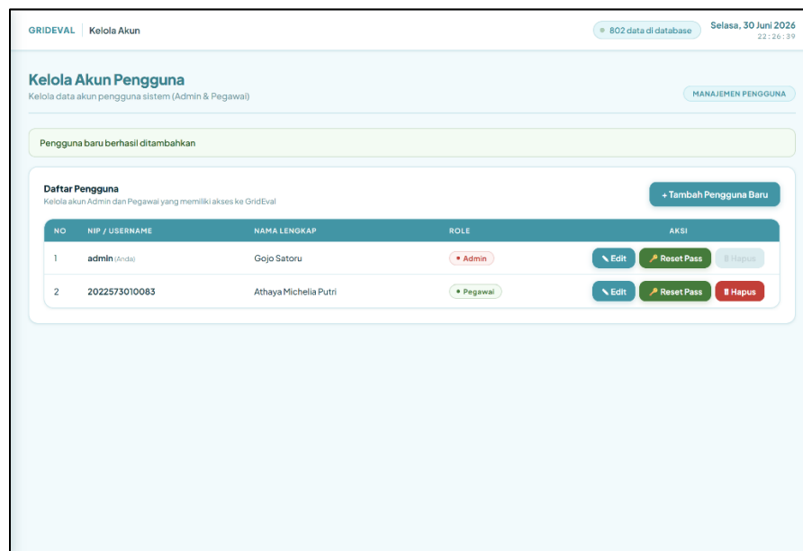
Gambar 4.11 Hasil Halaman Kelola Akun (Setelah Tambah Pengguna Baru)
